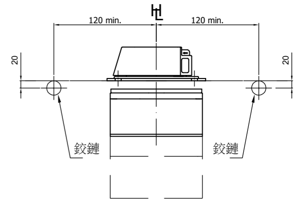
鉸鏈之距離
