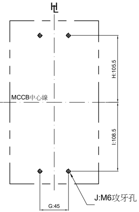
MCCB固定孔
